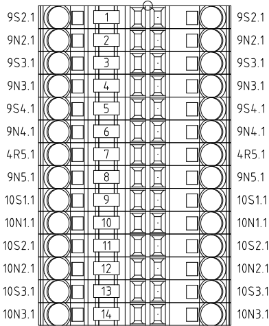
+QG - XZ2 ZONA 3 (9TR1)
