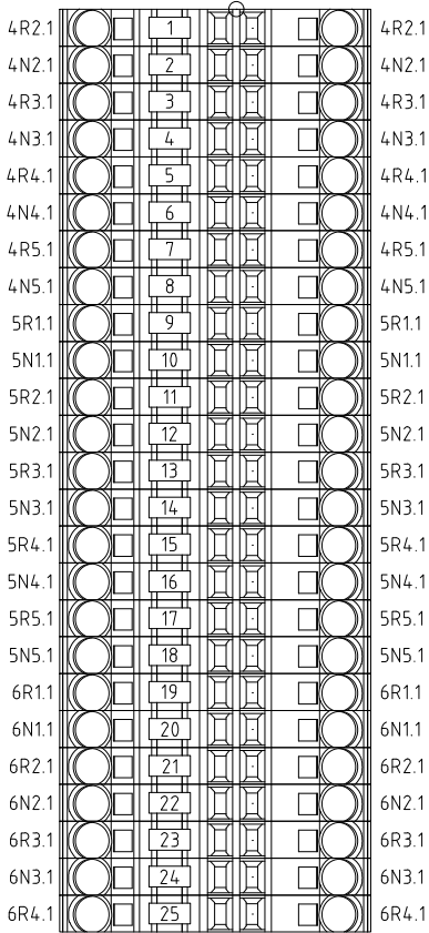
+QG - XZ1 ZONA 3 (4TR1)
