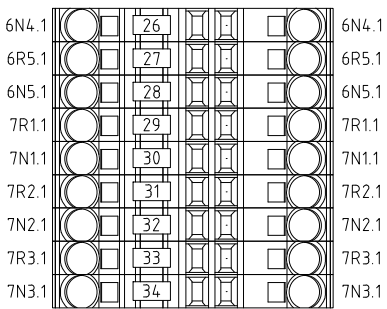
+QG - XZ1 ZONA 3 (4TR1)
